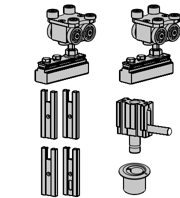
IN.15.550.3 Kit para painéis intermédios / Kit for middle panels / Kit para paneles intermedios.
