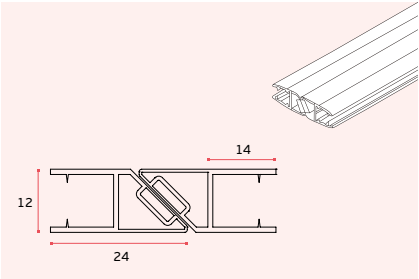
IN.15.999.C (2000mm) IN.15.999.C.L (2500mm) Vedante magnético para vidro 180° / 180° Magnetic PVC seals for glass / Sello magnetico para cristal 180°
