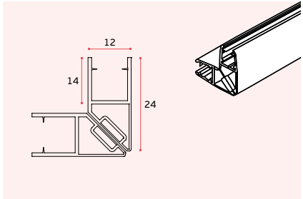
IN.15.999.B (2000mm) IN.15.999.B.L (2500mm) Vedante magnético para vidro 90° / 90° Magnetic PVC seals for glass / Sello magnetico para cristal 90°
