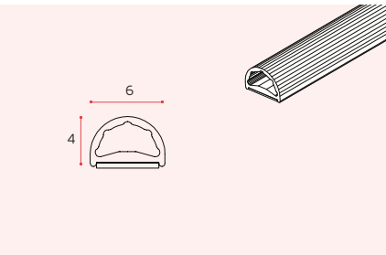
IN.15.995.E (12mt) Vedante para vidro / PVC seals for glass / Sellos para cristal
