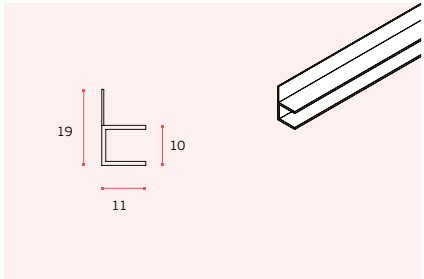
IN.15.997.F (2000mm) IN.15.997.F.L (2500mm) Vedante para vidro / PVC seals for glass / Sellos para cristal
