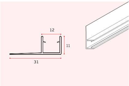
IN.15.999.F (2000mm) IN.15.999.F.L (2500mm) Vedante para vidro / PVC seals for glass / Sellos para cristal
