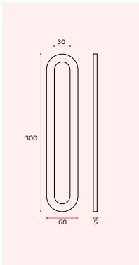
IMAGEM / IMAGE / IMAGEN: IN.16.562.A (x2)
