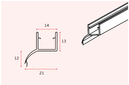
IN.15.999.H (2000mm) Vedante para vidro / PVC seals for glass / Sellos para cristal
