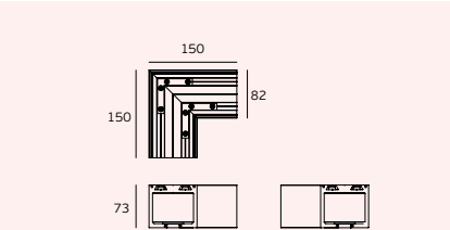
IN.15.553 União em "L" / "L" shaped union / Unión en "L".
