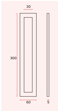
IMAGEM / IMAGE / IMAGEN: IN.16.558.A (x2)
