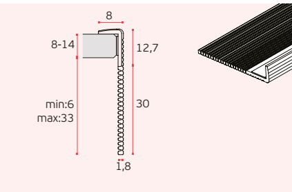
IN.15.995.F (3000mm) Vedante para vidro / PVC seals for glass / Sellos para cristal
