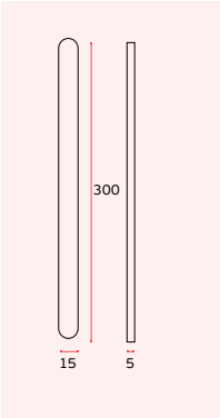
IMAGEM / IMAGE / IMAGEN: IN.16.556.A (x2)
