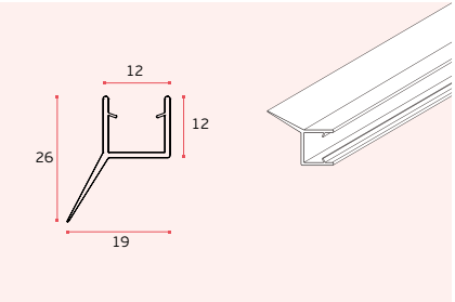
IN.15.999.A (2000mm) Vedante para vidro / PVC seals for glass / Sellos para cristal.
