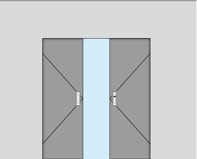
Vista interior >>> Kit de fechadura e conchas para portas duplas / Interior view >>> Flush handle and lock kit for double doors / Vista interior >>> Kit de cerradura y cazoleta para puertas dobles.
