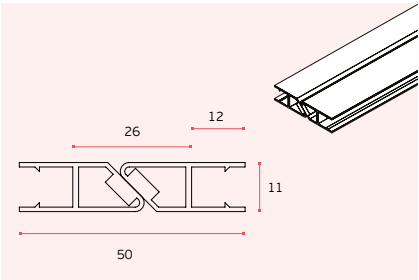
IN.15.997.C (2000mm) IN.15.997.C.L (2500mm) Vedante magnético para vidro / Magnetic PVC seals for glass / Sello magnetico para cristal
