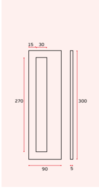
IMAGEM / IMAGE / IMAGEN: IN.16.560.A (x2)
