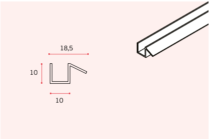
IN.15.997.J (2000mm) Vedante para vidro / PVC seals for glass / Sellos para cristal
