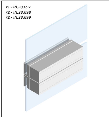
Aplicação para porta e bandeira em vidro. Caixas sobrepostas com pinça de vidro / Application for glass door and flag. Overlapping boxes with glass clamp / Aplicación para puerta y bandera de cristal. Cajas superpuestas con pinza para cristal /
