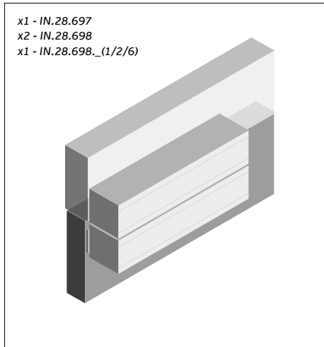
Aplicação para portas de madeira ou metálicas. Solução sobreposta no aro e porta com placas de compensação / Application for wooden or metal doors. Rim solution in the frame and door with compensating plates / Aplicación para puertas de madera o metal. Solución sobrepuesta en el marco y la puerta con placas compensadoras.
