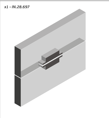
Aplicação para portas de madeira ou metálicas. Solução embutida no aro e porta / Application for wooden or metal doors. Built-in solution in the frame and door / Aplicación para puertas de madera o metal. Solución empotrada en el marco y la puerta /
