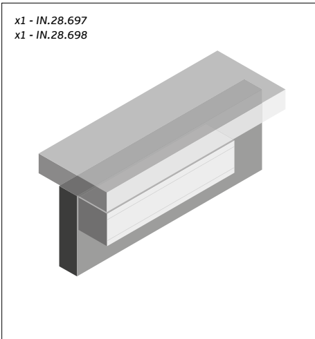
Aplicação para portas de madeira ou metálicas. Solução sobreposta na porta e receptor embutido no tecto ou aro / Application for wooden or metal doors. Box overlapped in the door and receiver embedded in the ceiling or frame / Aplicación para puertas de madera o metal. Caja sobrepuesta en la puerta y receptor empotrado en el techo o el marco.
