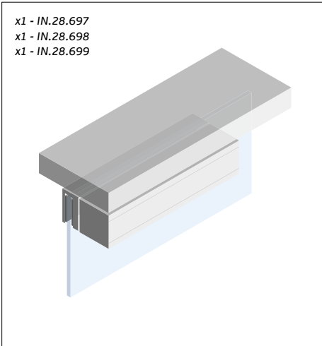
Aplicação para portas de vidro. Caixa sobreposta na porta e recetor embutido no teto ou aro / Application for glass doors. Box overlapped in the door and receiver embedded in the ceiling or frame / Aplicación para puertas de cristal. Caja sobrepuesta en la puerta y receptor empotrado en el techo o el marco.
