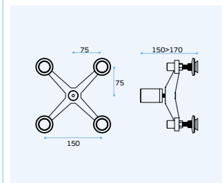
IN.82.001 Suporte para vidro com acessórios / Glass connector with accessories / Soporte para cristal con accesorios.
