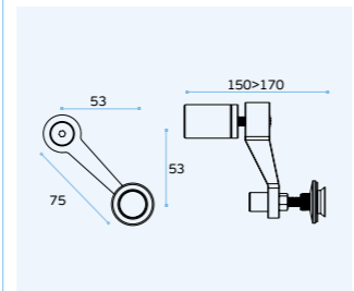
IN.82.004 Suporte para vidro com acessórios / Glass connector with accessories / Soporte para cristal con accesorios.
