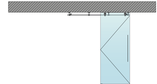
(B) FIXAÇÃO AO TECTO / FIXED AT CEILING / FIJO AL TECTO CARRIL / RAIL 1900mm
