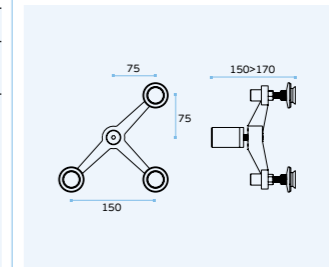
IN.82.006 Suporte para vidro com acessórios / Glass connector with accessories / Soporte para cristal con accesorios.
