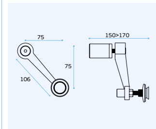
IN.82.003 Suporte para vidro com acessórios / Glass connector with accessories / Soporte para cristal con accesorios.
