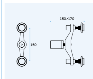
IN.82.005 Suporte para vidro com acessórios / Glass connector with accessories / Soporte para cristal con accesorios.
