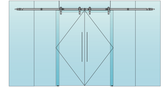
(C) FIXO NO VIDRO / FIXED AT GLASS / FIJA EN Cristal
