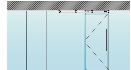
(D) FIXAÇÃO AO TECTO E VIDRO / FIXED AT CEILING AND GLASS / FIJO EN TECTO Y CRISTAL CARRIL / RAIL 1900mm
