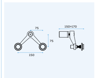
IN.82.002 Suporte para vidro com acessórios / Glass connector with accessories / Soporte para cristal con accesorios.
