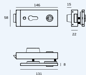
IMAGEM / IMAGE: IN.20.360 IN.00.037.SR IN.19.S22.30.30
